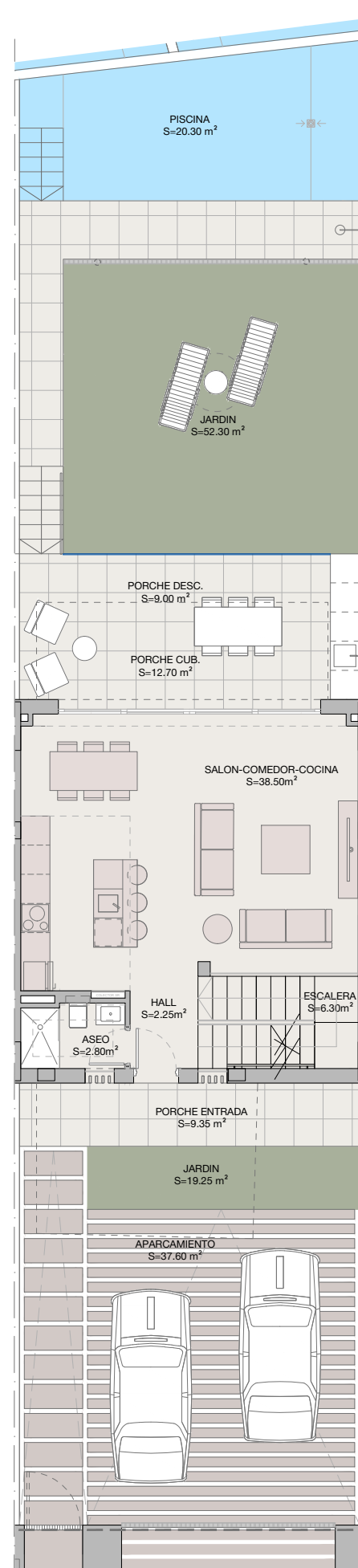
planta baja
