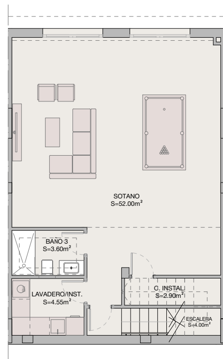
planta sotano
