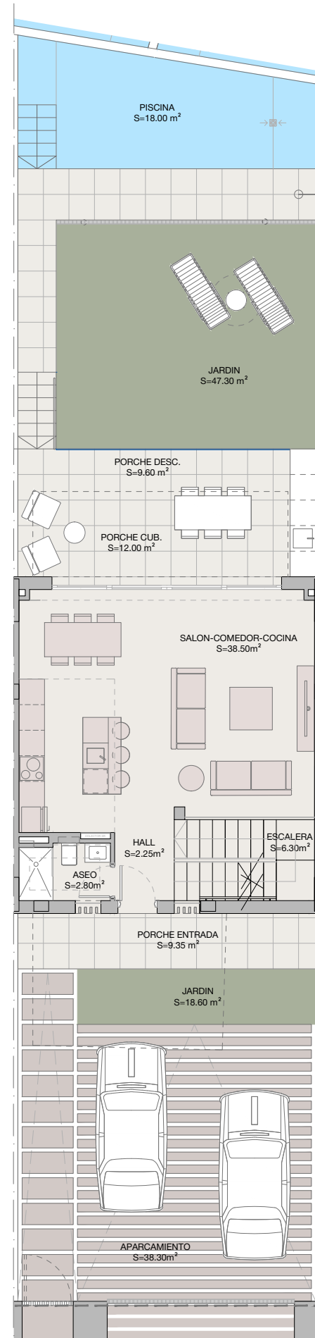
planta baja
