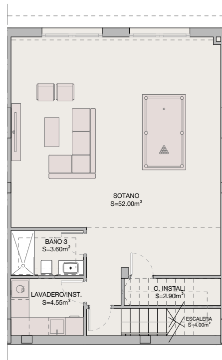
planta sotano
