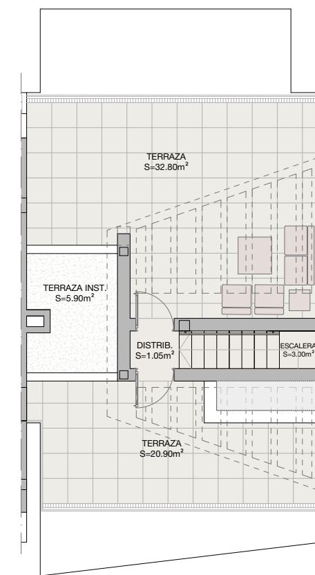
planta solarium
