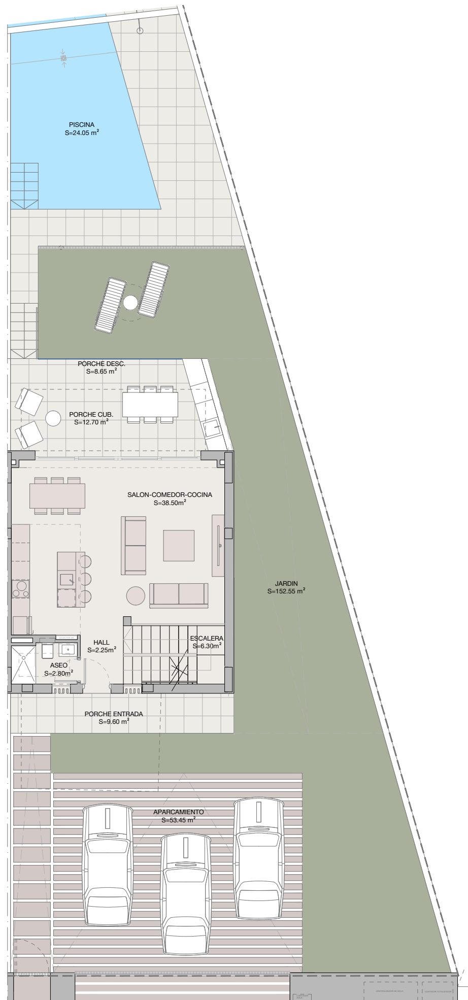
planta baja
