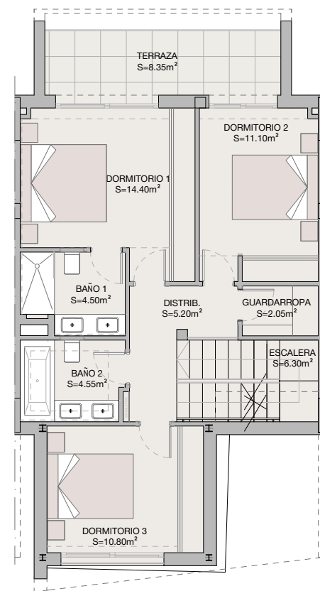
planta primera
