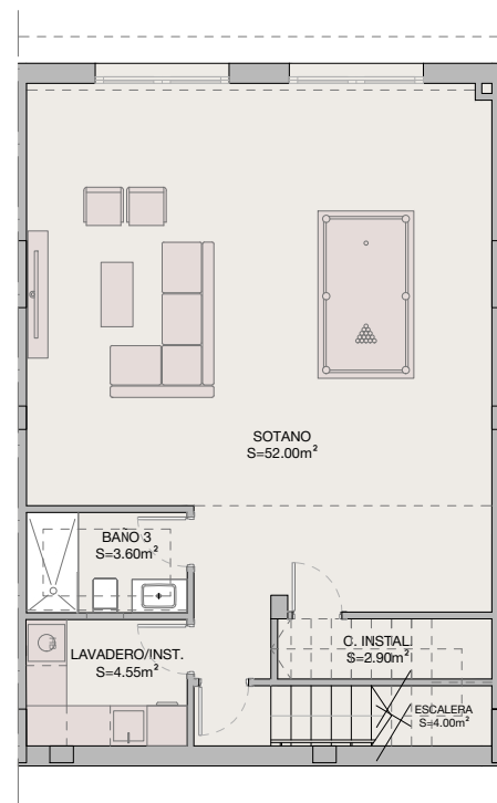
planta sotano
