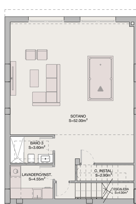
planta sotano
