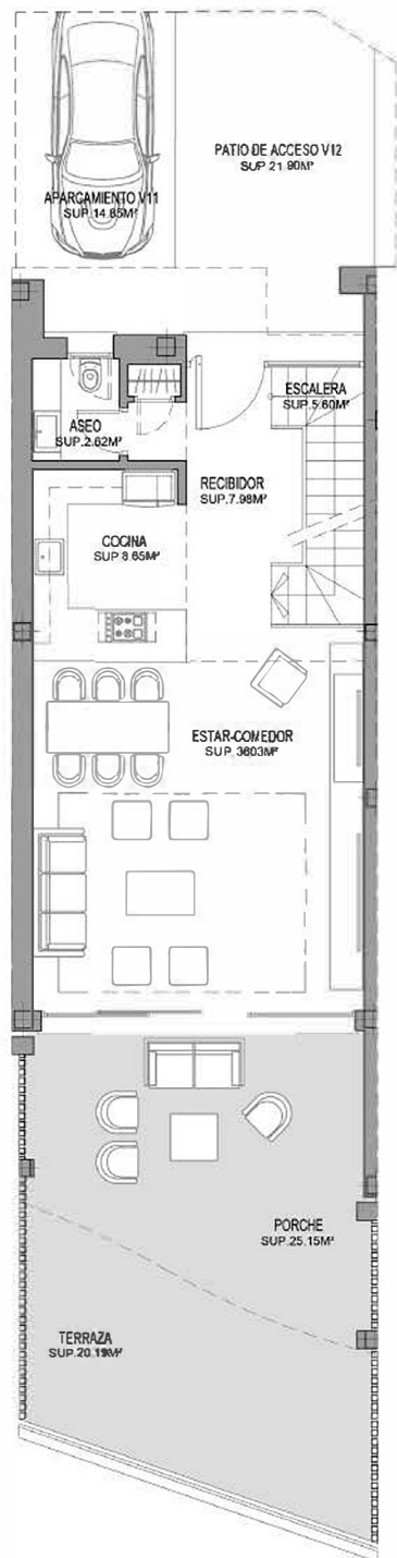
Planta Baja
