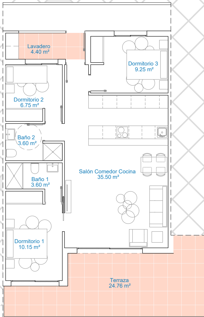
PLANTA PRIMERA
